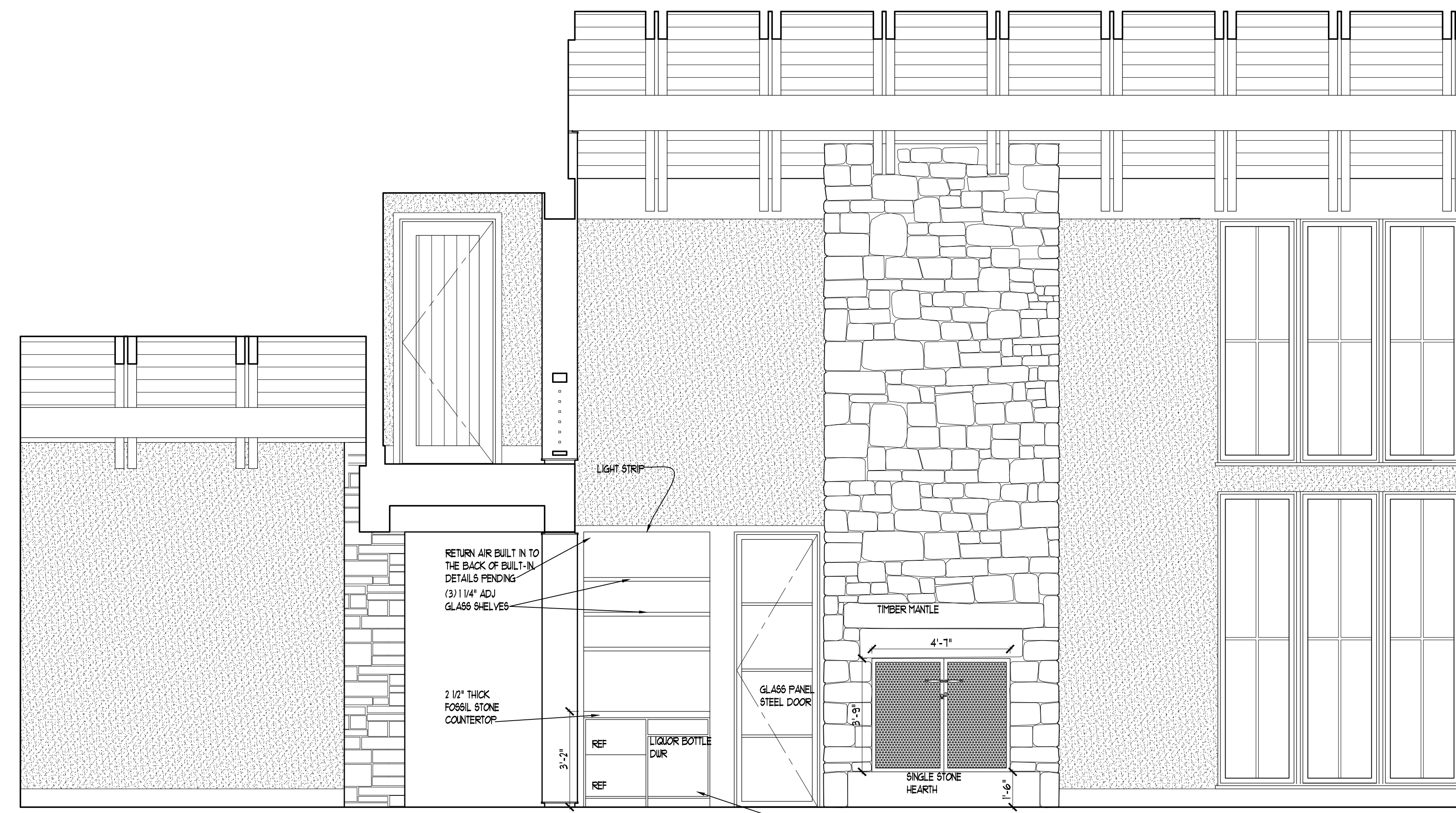
44 A13 ENTRY -101- WEST SCALE: 3/8" = 1'-0"
